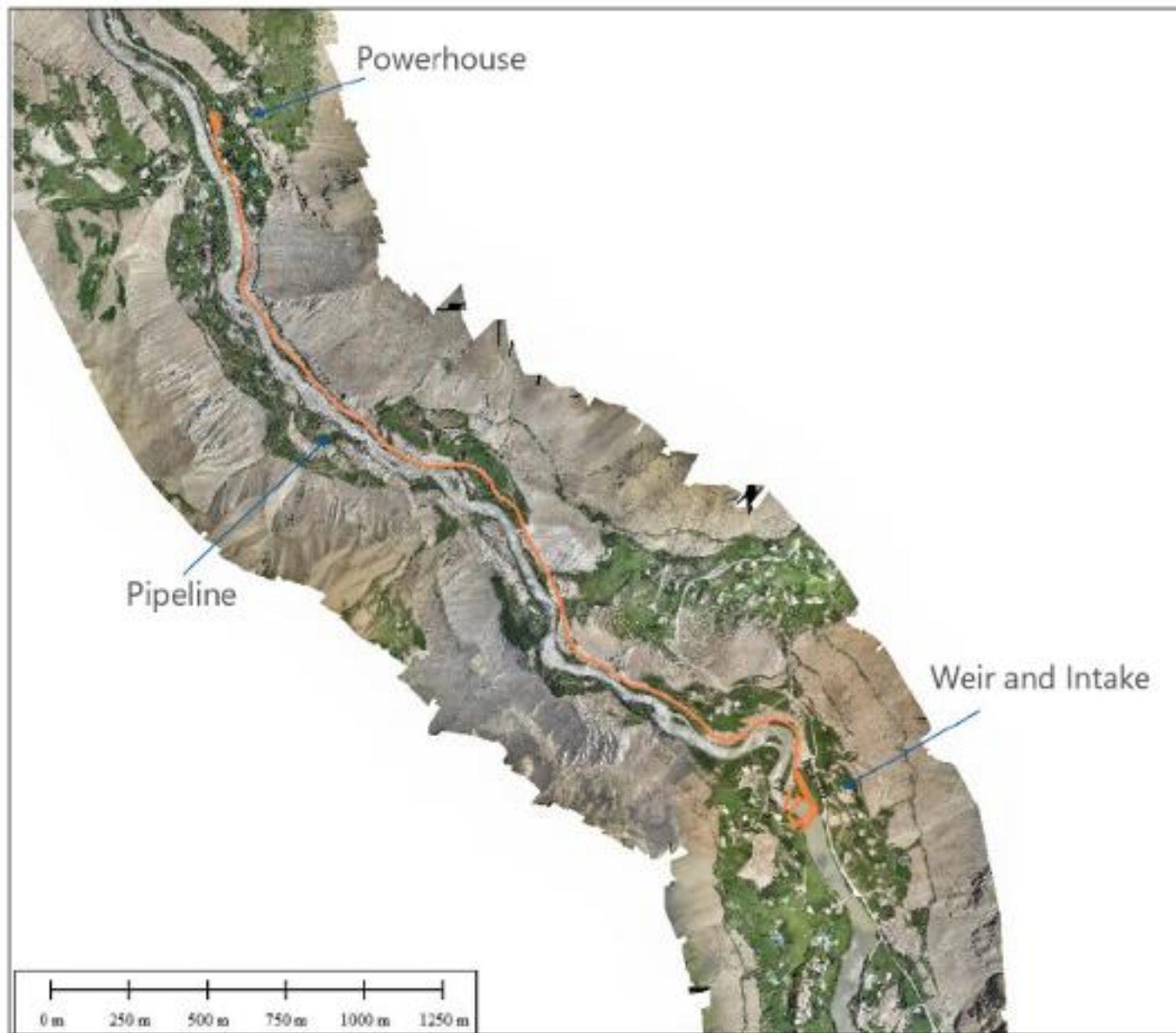
Иллюстрация 3 – Схема расположения проекта Себзорской ГЭС согласно обновленному рабочему варианту ТЭО (Фихтнер 2021 г.). Трубопровод протяженностью 3 км между водозабором и электростанцией будет проложен по дороге на правом берегу реки Шохдара. От подстанции рядом с электростанцией 18-километровая линия электропередачи в 110 кВ пройдет к новой подстанции в главном операционном центре Компании Памир Энерджи в г. Хороге, рядом с Хорогской ГЭС.
